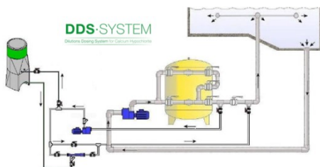
VENTURI
